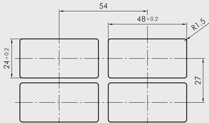
Einbaumaße Typen LX...
